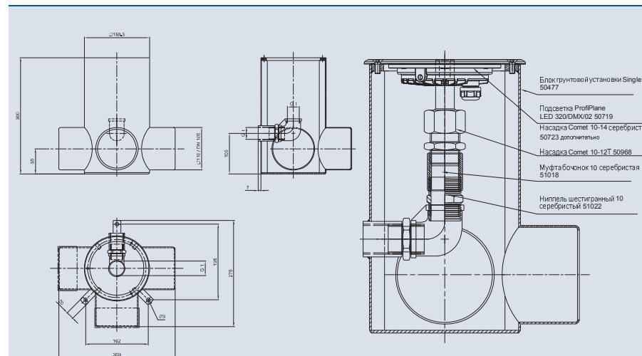
Блок грунтовой установки Single
