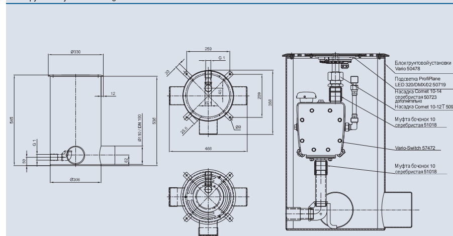
Блок грунтовой установки Single
