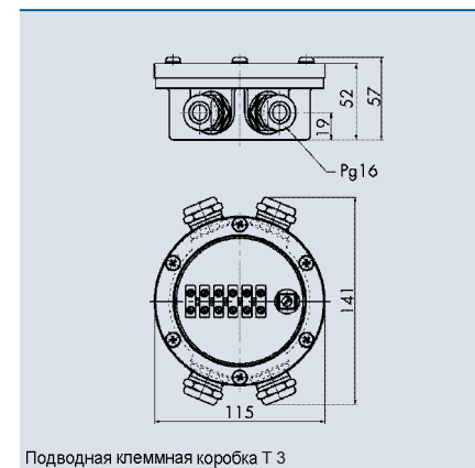
Подводная клеммная коробка Т 3
